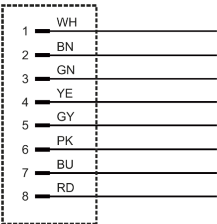
Schaltplan
