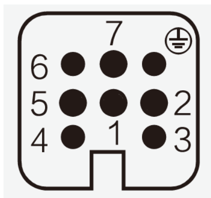
Pinbelegung
