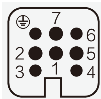
Pinbelegung
