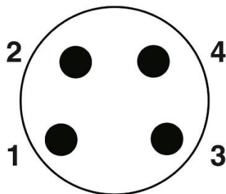
Polbild M8-Stecker, 4-polig, A-kodiert, Ansicht Stittseite
