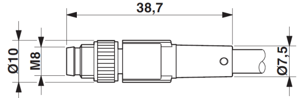
Stecker M8 x 1, gerade
