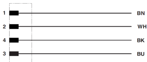
Kontaktbelegung des M8-Steckers
